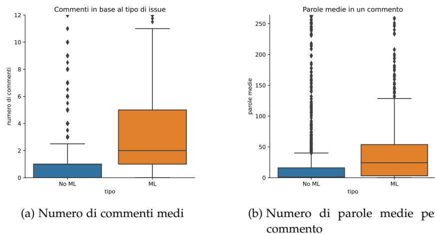
Figura 2.5: Livello di discussione in base al tipo
