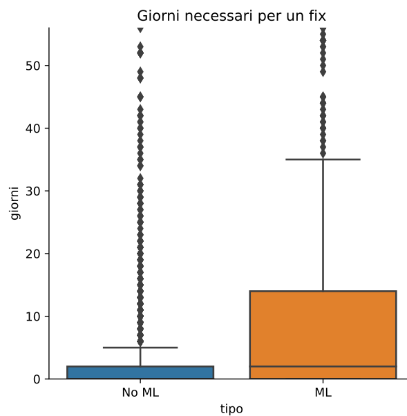
Figura 2.6: Giorni necessari per il fix
